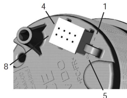
Rückansicht VL Flex 52 Tyco / Hirschmann 8-Pol MQS Stecker
